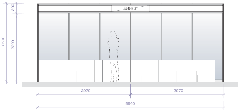
立面図
