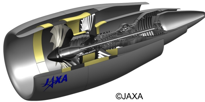
より環境にやさしいジェットエンジン [提供・JAXA]
