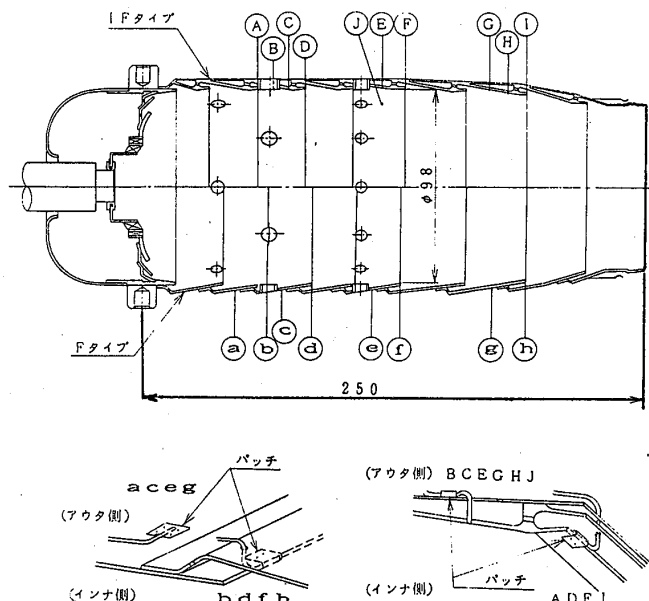
図4. 供試燃焼器と熱電対埋込み位置、方法。
