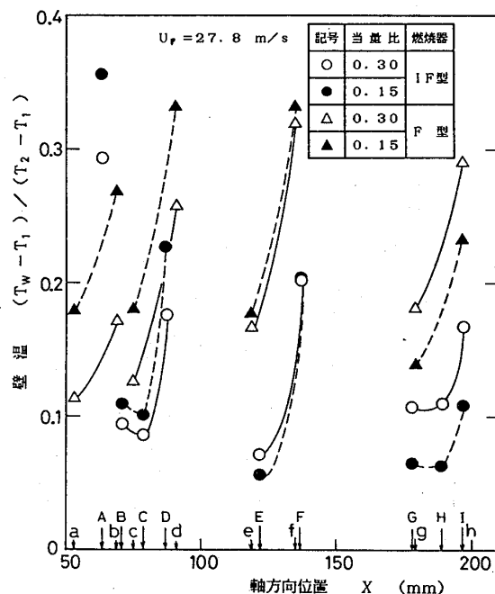
図5. 壁温分布
