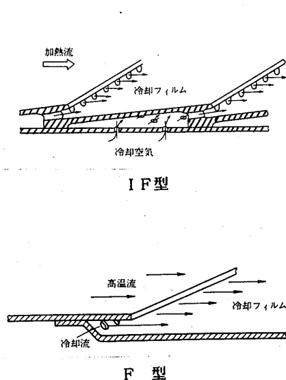
図3. 冷却構造
