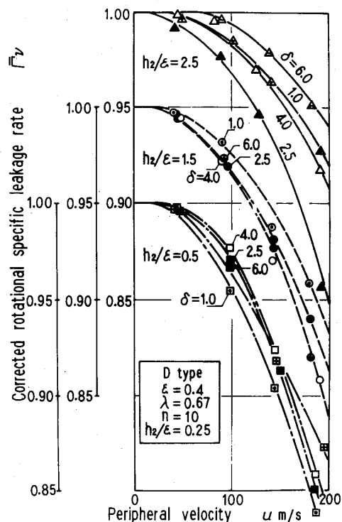
図7 絞り片厚さの影響
