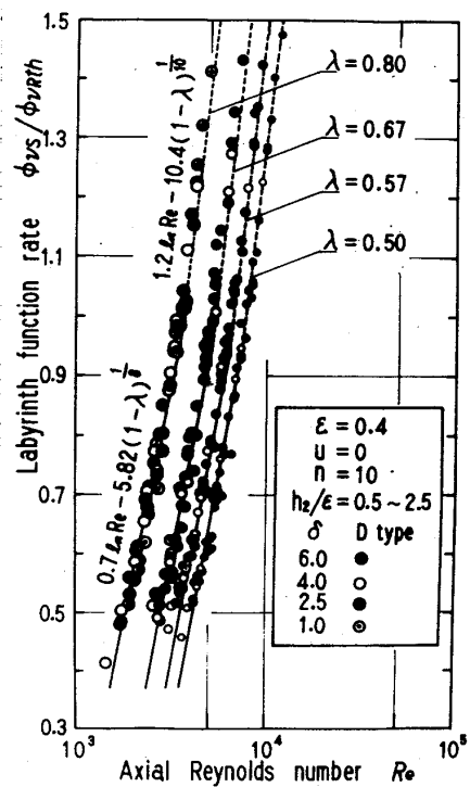
図4 \phi_{vs}/\phi_{vrtk} と Re の関係
