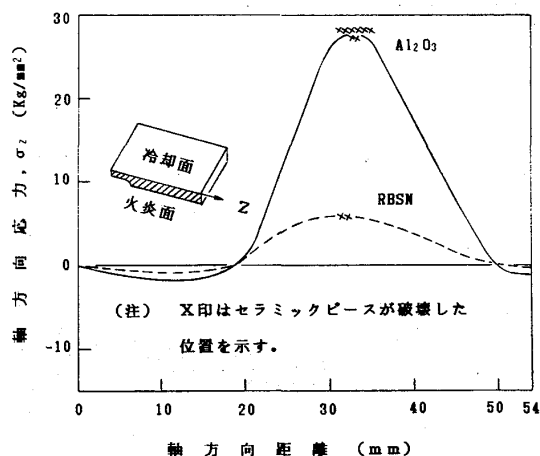
図6 軸方向応力分布と破壊位置
