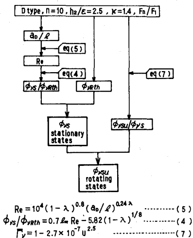
図13 予測計算の流れ図
