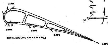
図2 E 3 (ENERGY EFFICIENT ENGINE) 計画の冷却タービン
