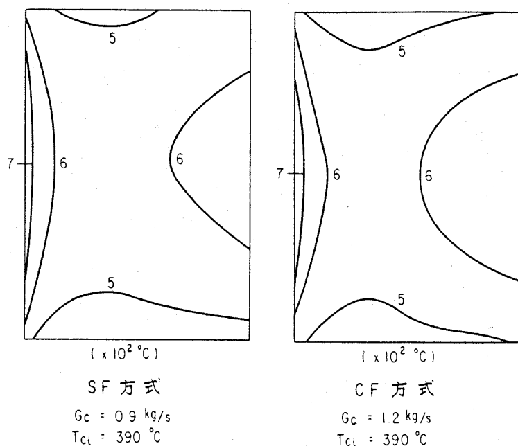
図 4 浸出無し空冷翼面温度分布計算例 ( \bar{T}_{GO1} = 1000 °C, G = 2.6 kg/s)
