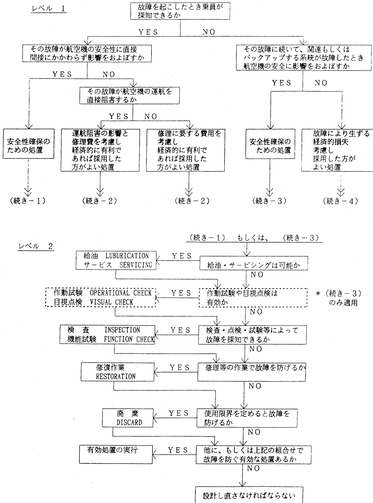
図2 MSG-3による整備要目の分析
