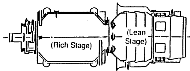
図11 RBQQLB 燃焼器 (4)
