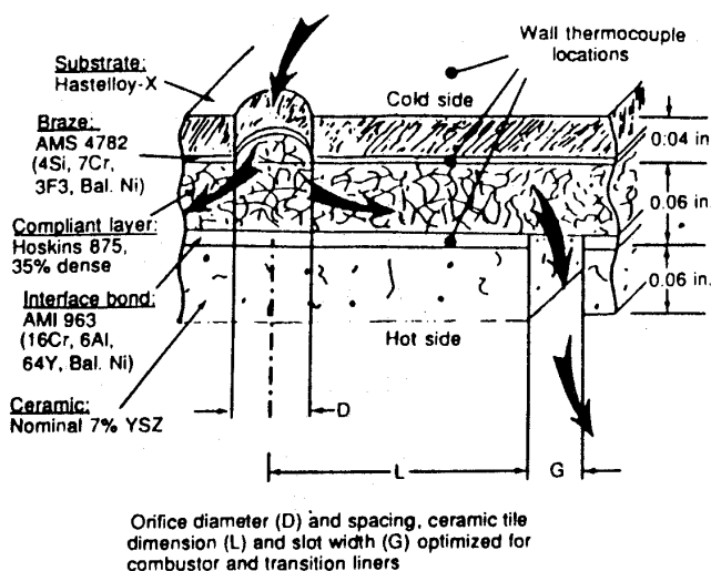
図4 コンプライアントメタルセラミックライナ (8)
