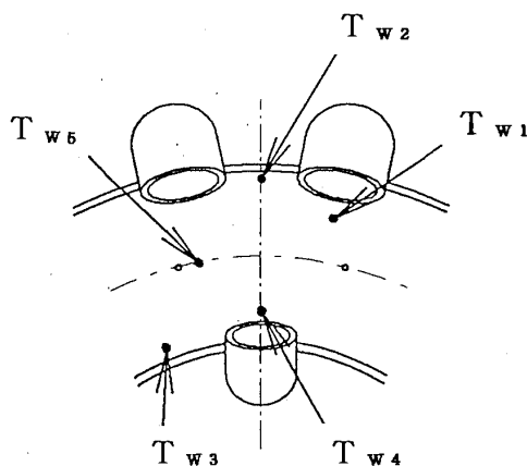
(b) 下流側から見た熱電対取り付け位置
