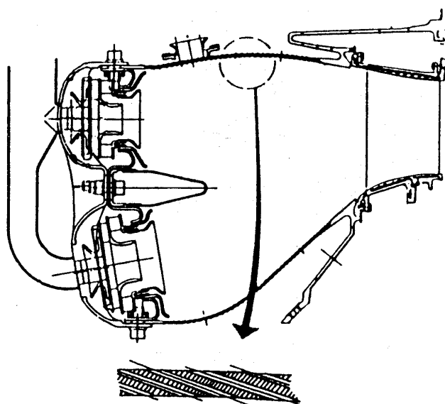
図3 GE 90 燃焼器 (7)
