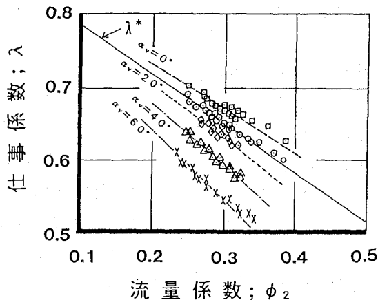
図 20 仕事係数
