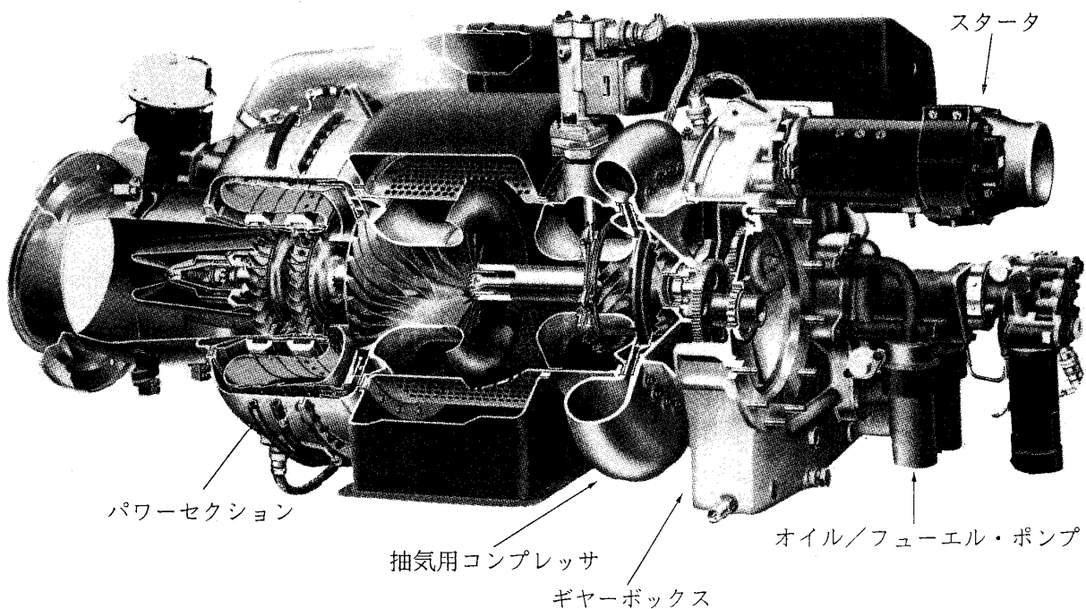
図 1 APU 131-9 構造図
