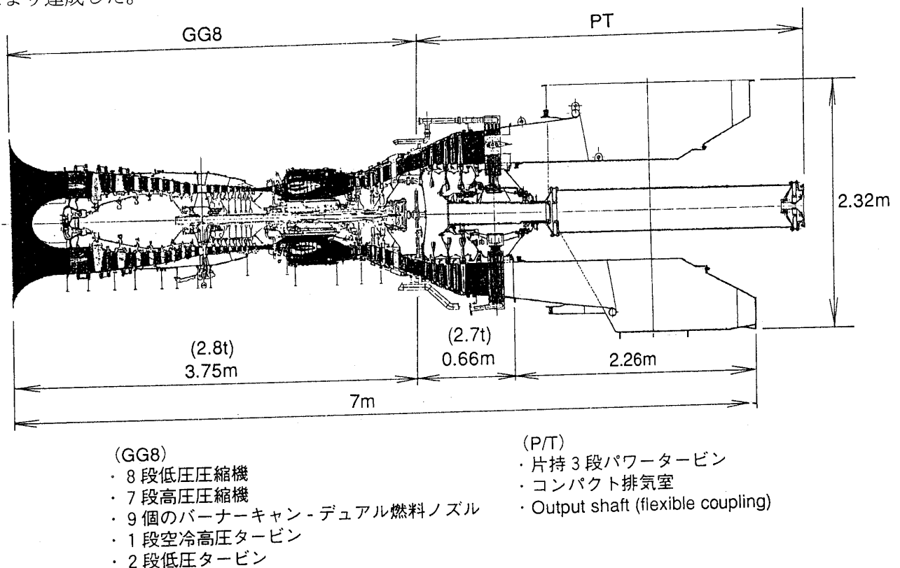
図 3.1.1 MFT8 ガスタービン断面図
