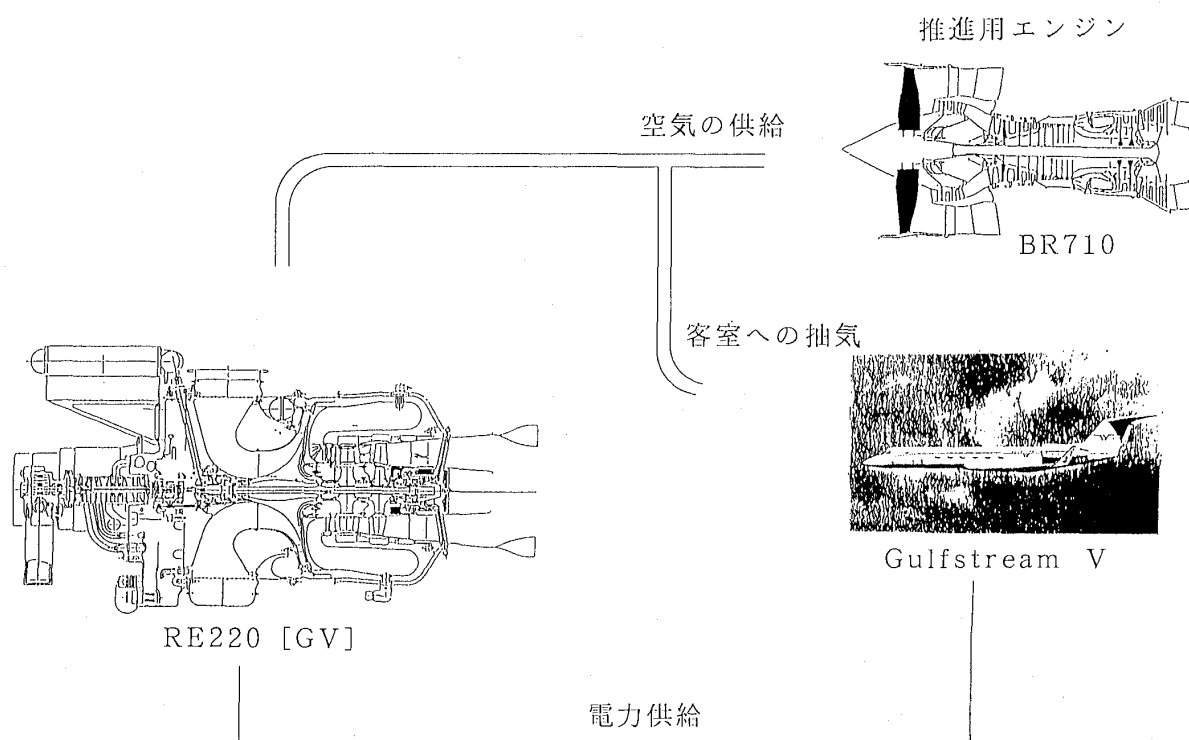
図4 APUの機能
