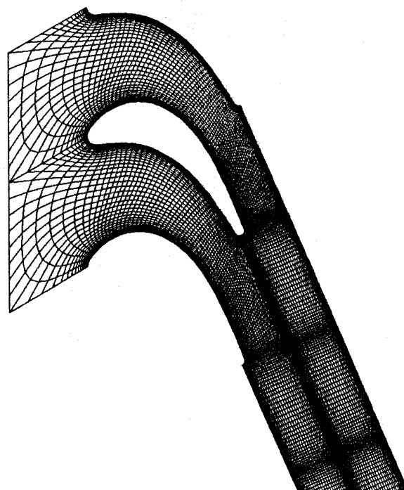
図5 計算格子
