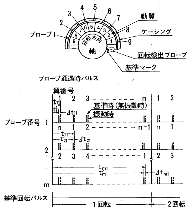
図1 計測原理
