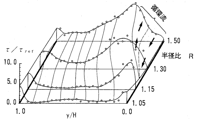
図5 剪断応力分布
