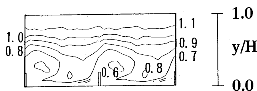
(c) 半径比 R=1.80
