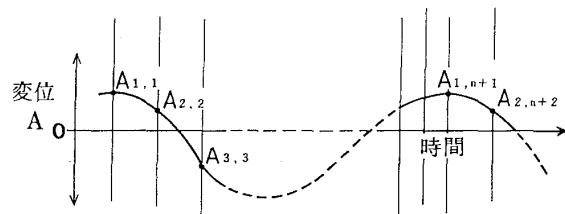
(b) 動翼 B_1 の振動波形
