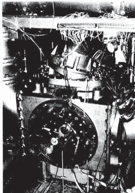
写真2 熱サイクル試験装置本体部の外観
