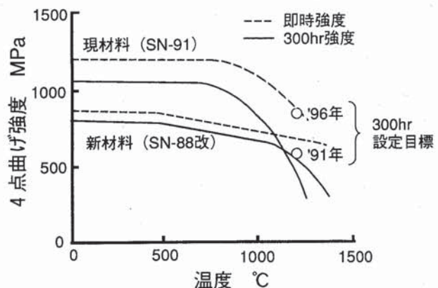
図4・8 材料強度特性
