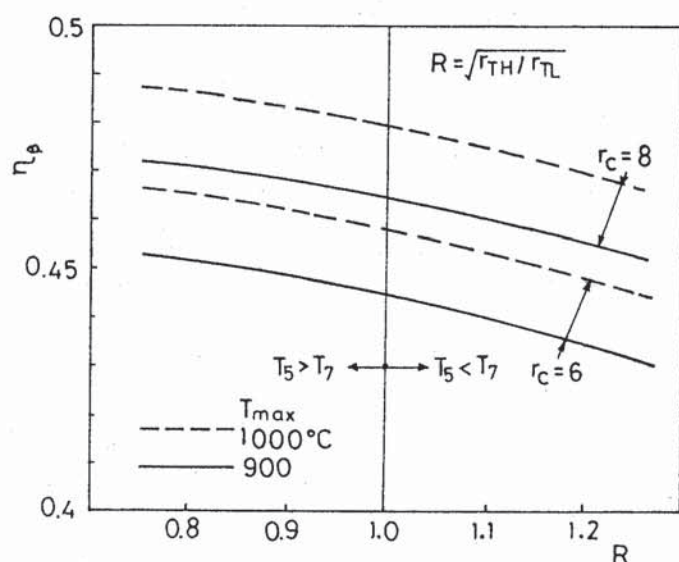
図7 タービン圧力比による性能の相違
