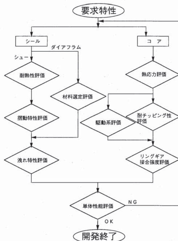
図6・3 熱交換器開発プロセス
