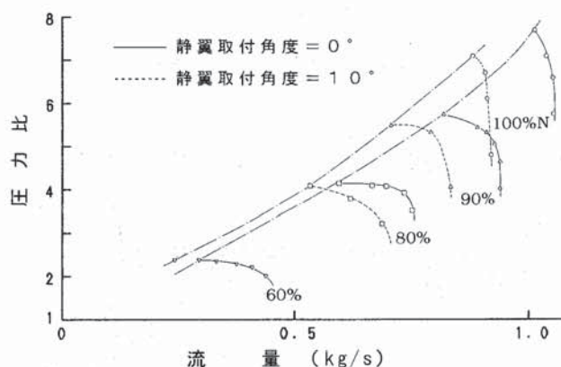
図14 軸流+遠心圧縮機の性能
