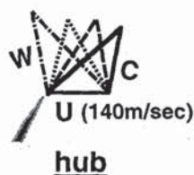
図 3・10 インペラ入口速度三角形
