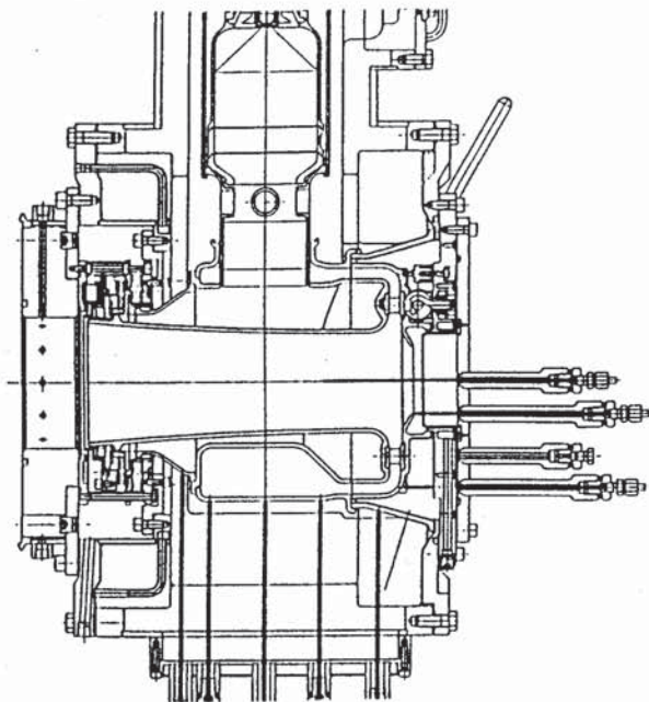
図4・14 静止部品組合せ試験装置
