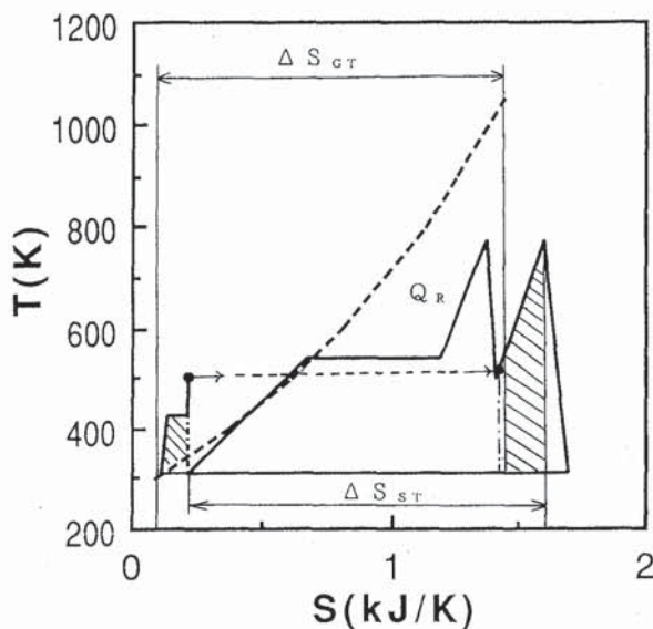
図2 2重圧サイクル
