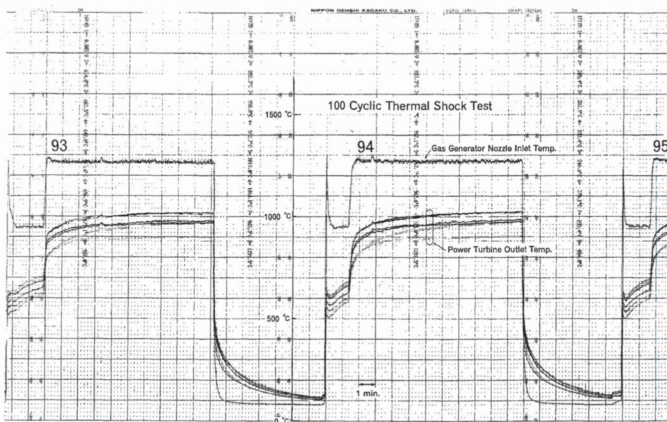
図5 熱衝撃試験時の温度記録
