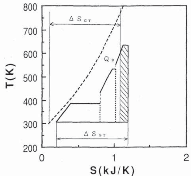
図3 混圧サイクル
