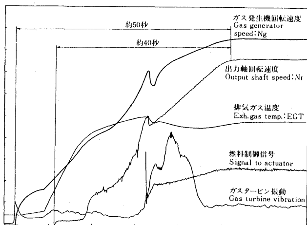
図5 有負荷始動チャート
