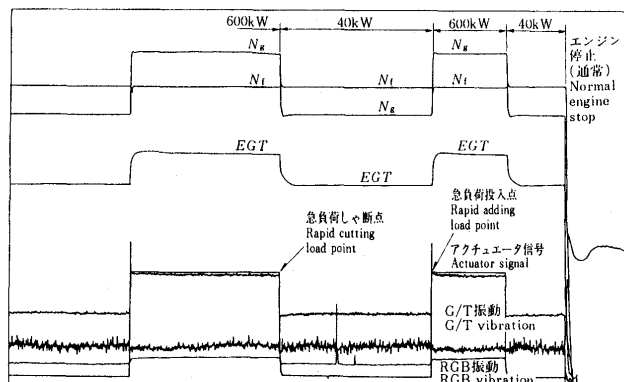
図7 急負荷変動試験
