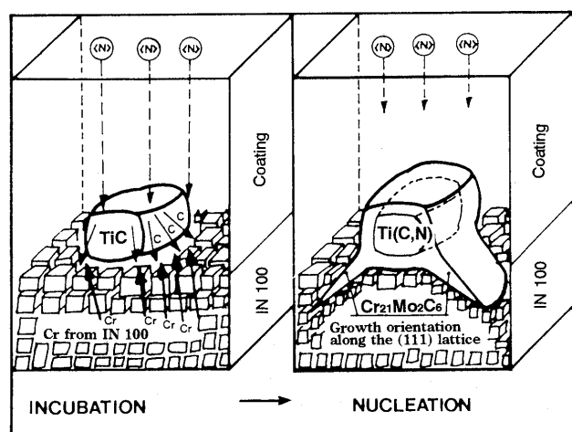
図27 針状析出物の成長モデル (66)
