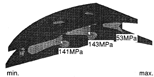
図 18 熱衝撃試験条件での応力分布
