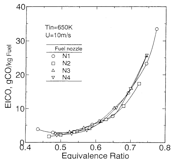
図4 DS バーナにおいて各ノズルを用いたときの CO 排出特性
