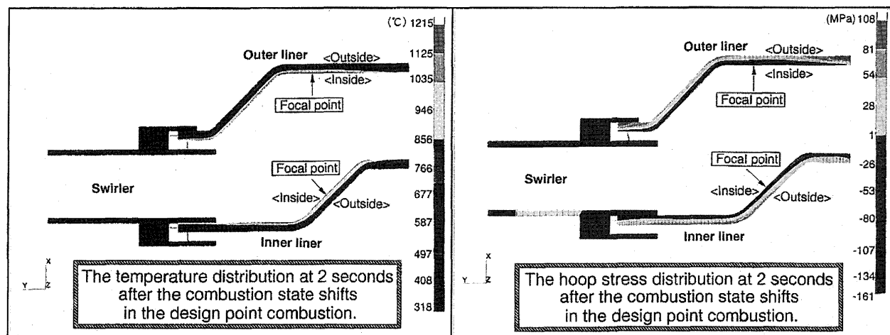
(A)非定常熱伝導解析結果(アイドル→定格 2 sec 後)
