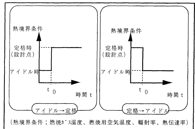
図3 熱境界条件の変化
