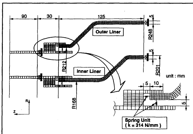
図2 複合材ライナの熱応力解析モデル
