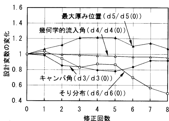
図9 最適化による設計変数の変化
