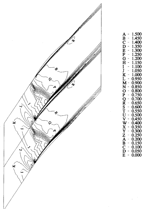
図8 初期形状解析結果（マッハ数分布）
