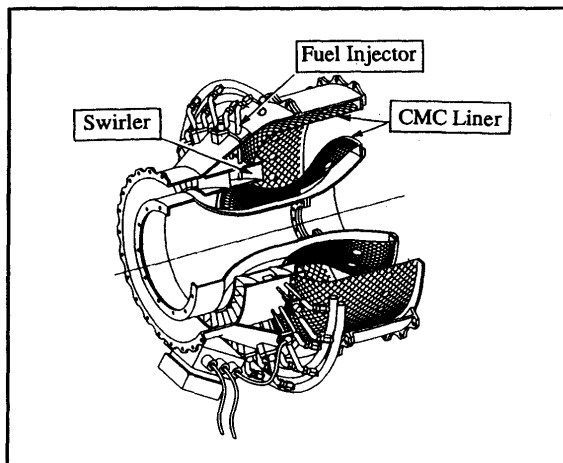
図1 AMG 燃焼器の構成概念図
