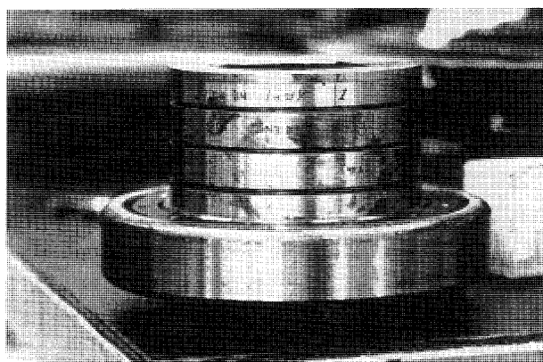
図2 輪バネを使った軸受構造 (もう1個の軸受が対称位置に組付けられる)
