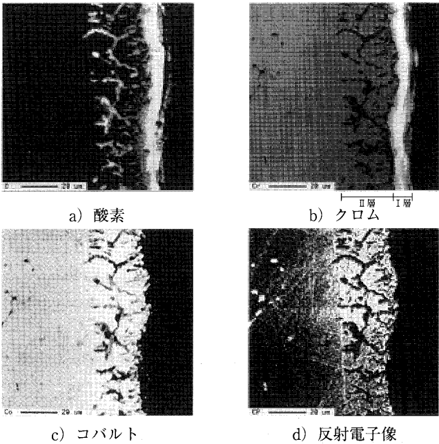
図 20 EPMA 写真
