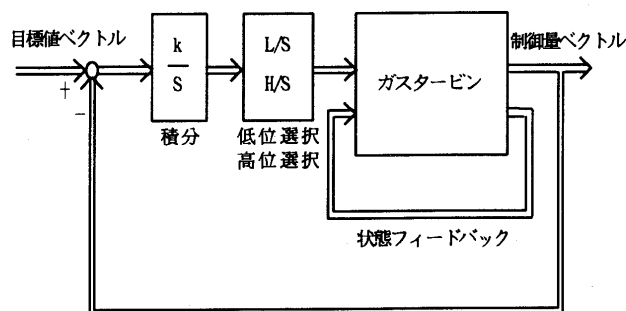
図5 ガスタービンの IESF 制御方式
