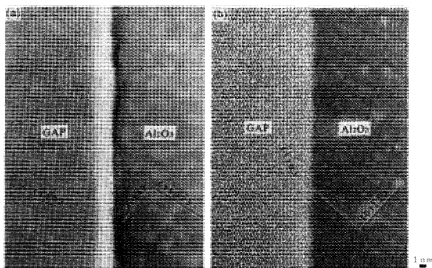
図10 \text{Al}_2\text{O}_3/\text{GAP} 系焼結複合材料の結晶粒界および \text{Al}_2\text{O}_3/\text{GAP} 系MGC材料の界面のHRTEM像
