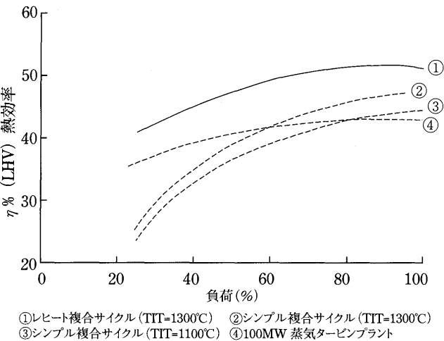
図 15 コンバインドサイクル部分負荷特性
