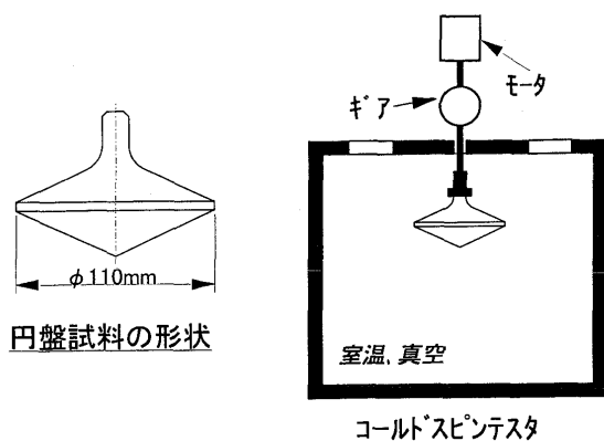
図8 円盤形状試料とコールドスピントスタの概要図
