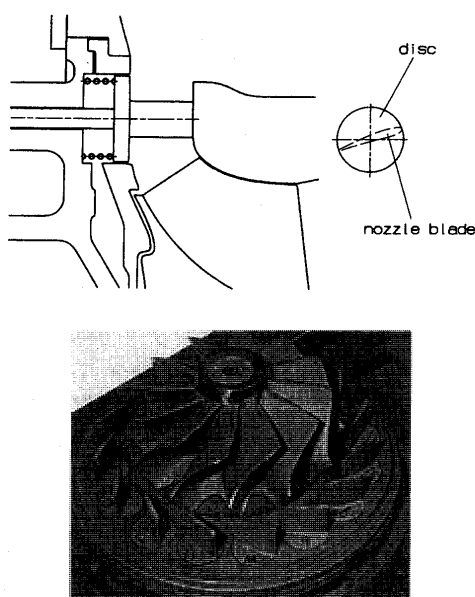
図6 斜流タービンと可変ノズル羽根の組合せ (14)
