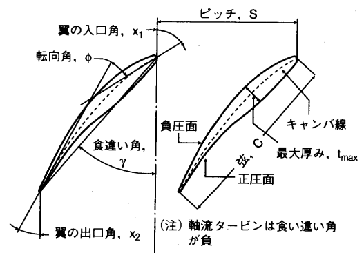
図 18 圧縮機翼列幾何形状
