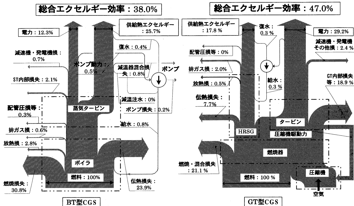
図6 CGSの総合エクセルギー効率
