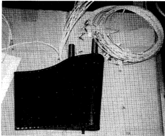
図 12 試験翼
