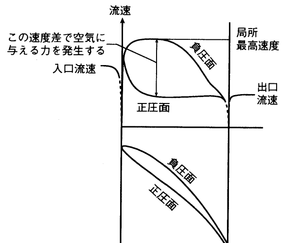
図 19 軸流圧縮機翼列の翼面速度分布
