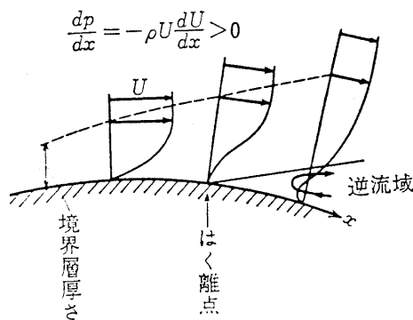
図 17 正の圧力勾配にある境界層
