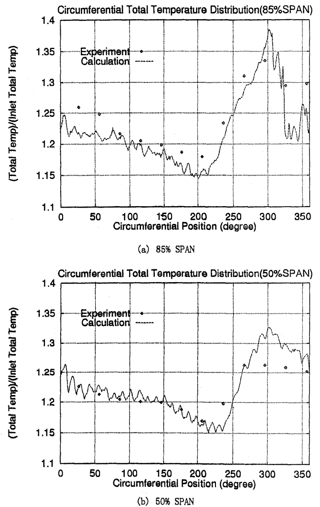
図3 ファンの下流の全温分布
