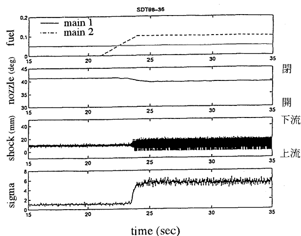
図 18 無制御状態での燃焼振動
