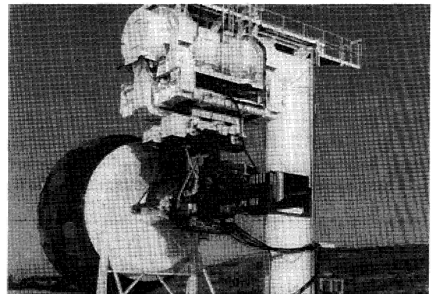
図 31 試作エンジン騒音試験 (Huknall)
