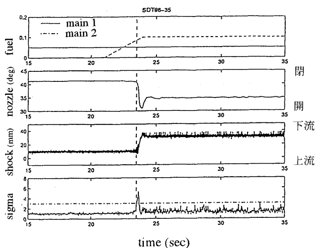
図 19 燃焼振動制御試験結果
