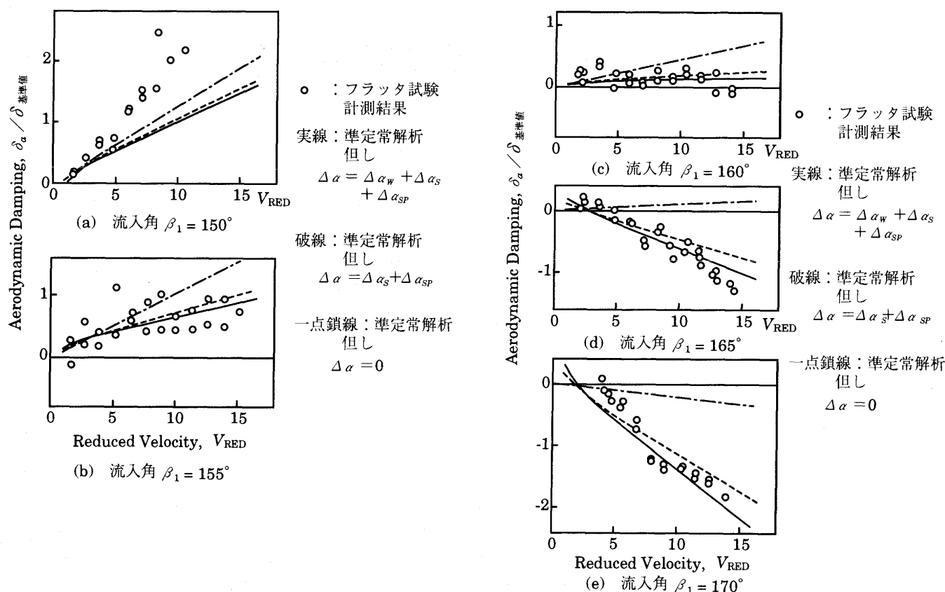
図7 準定常解析結果とフラッタ試験結果との比較
