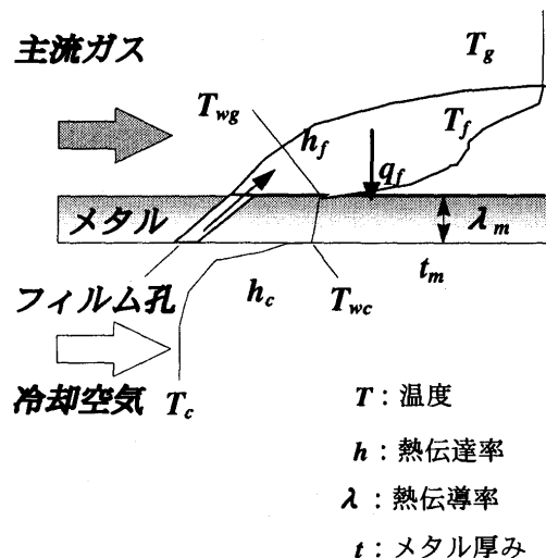
図2 フィルム冷却のある場合
