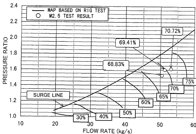
図3 ファン部のエンジン試験結果 (M 2.5)
