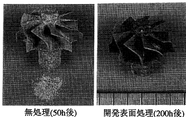
図5 950℃、排気ガス中酸化後のタービンホイール外観
