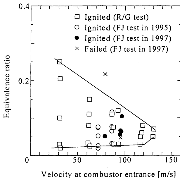
図 17 試験に使用した小型燃焼器の着火特性
