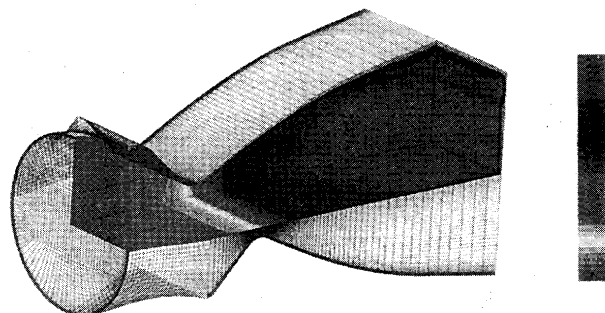
図16 3次元粘性解析結果
