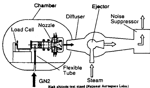
図19 ターボ域ノズル空力試験装置
