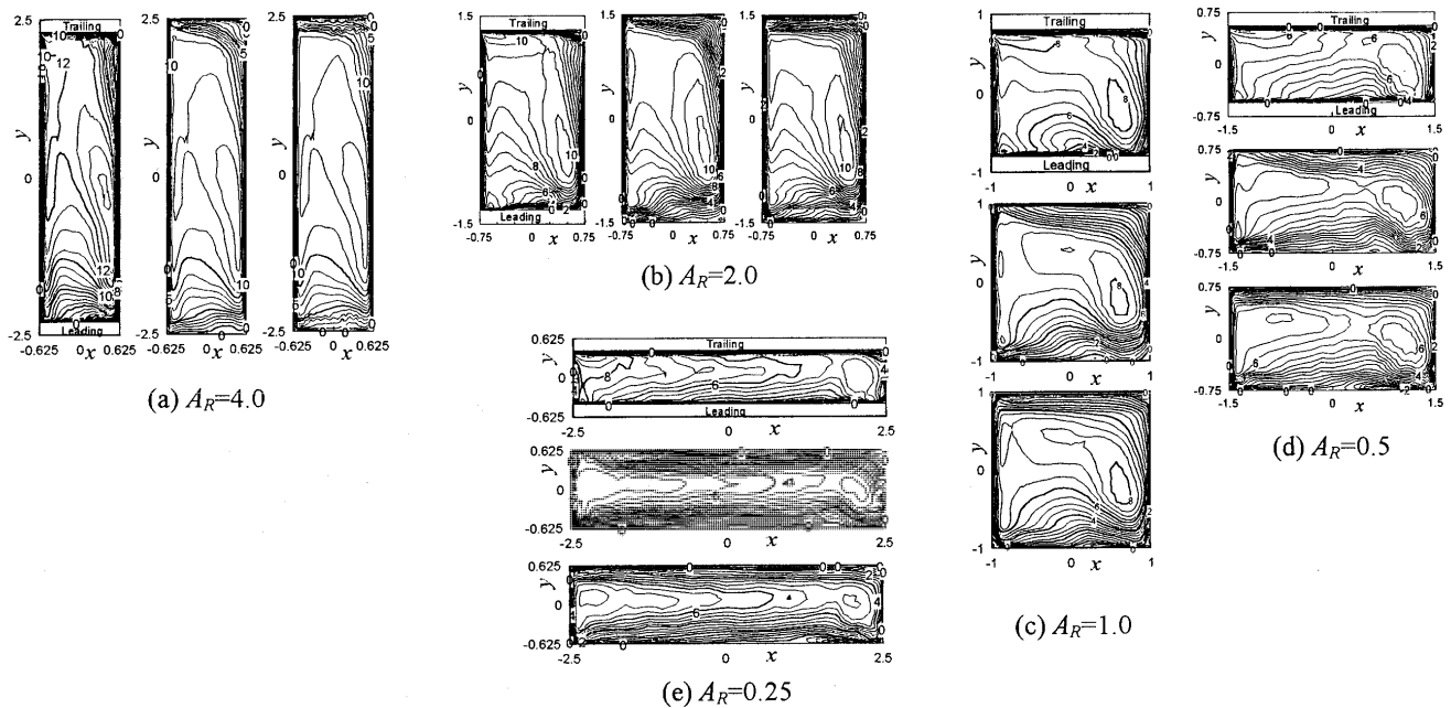
図 6 流れ方向 3 ケ所での \xi - \eta 断面内時間平均主流方向速度 \bar{w} 分布 ( 60^\circ リブ, Ro_\tau=1 の場合。他の説明は図 2 に同じ)
