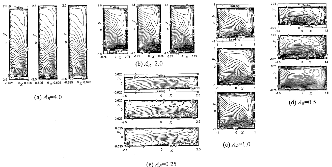
図 7 流れ方向 3 ケ所での \xi - \eta 断面内時間平均温度 \bar{\theta} 分布 ( 60^\circ リブ, Ro_\tau=1 の場合。他の説明は図 2 に同じ)
