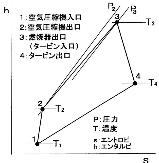
図2 ガスタービンサイクル
