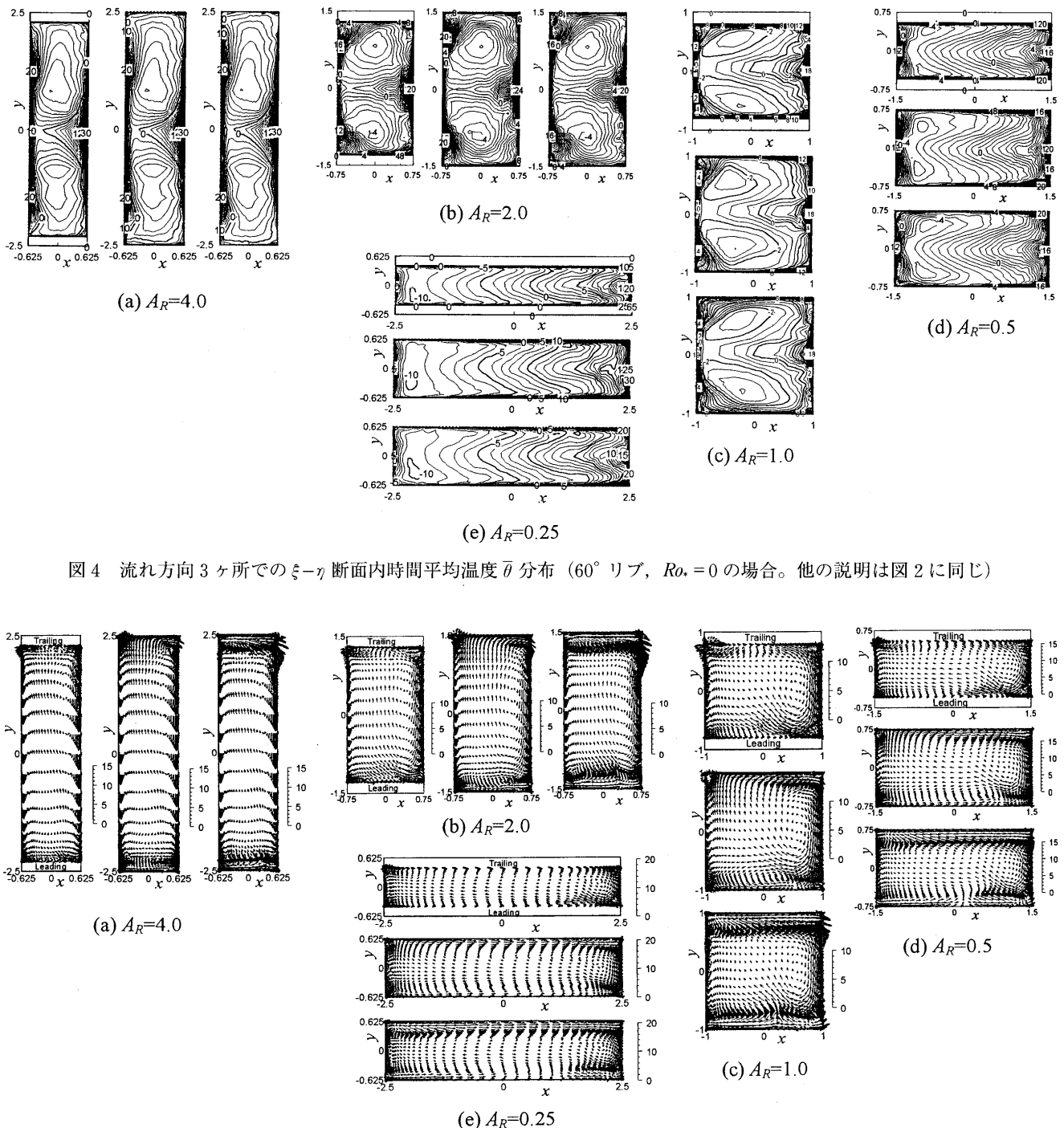
図5 流れ方向3ヶ所での \xi - \eta 断面内時間平均速度ベクトル図 ( 60^\circ リブ, Ro_\tau = 1 の場合。他の説明は図2に同じ)
