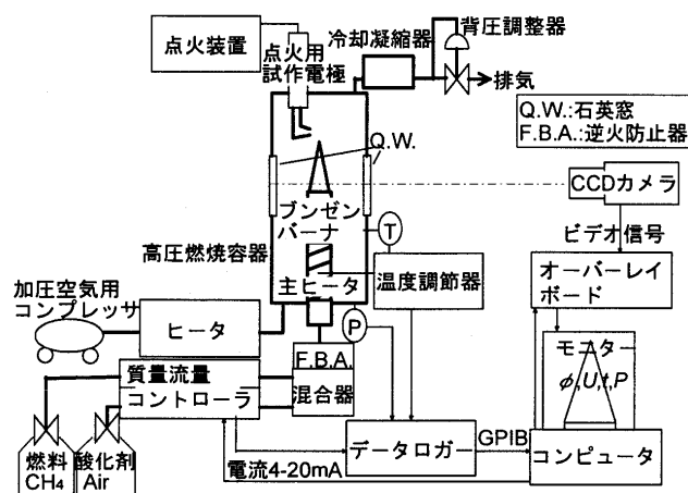
図1 実験装置
