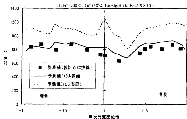
図11 静翼メタル温度分布(設計点)
