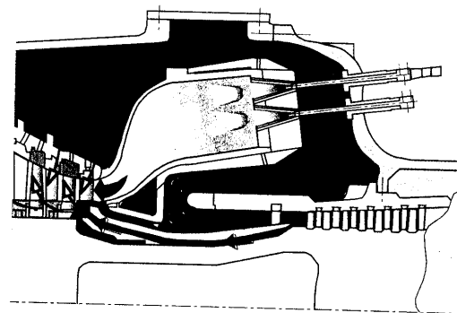
(a) 燃焼器構造(ABB)
