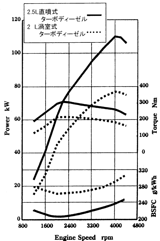
図10 2.5L直噴ターボディーゼルエンジン性能
