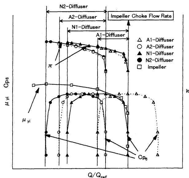
図10 インペラとディフューザの組合わせ (概念図)
