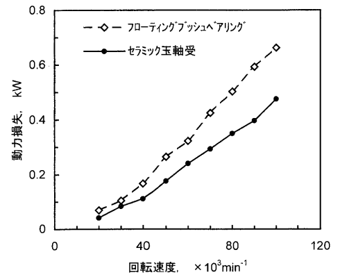
図3 動力損失
