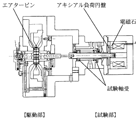
図1 試験装置
