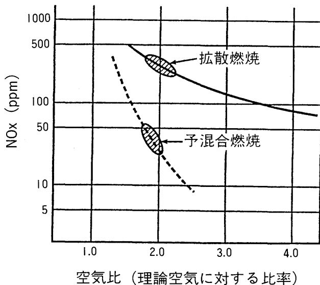
図 24 拡散燃焼と予混合燃焼の特徴 (6)
