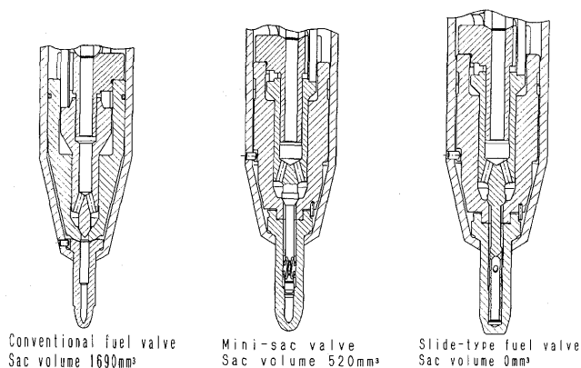
図8 燃料弁構造の比較
