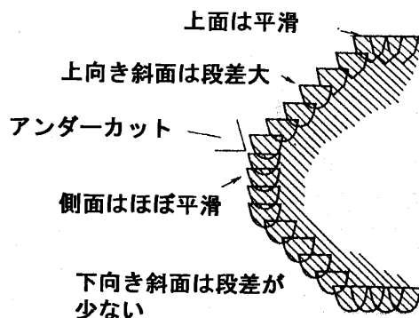
図8 光造形法による表面段差のイメージ図
