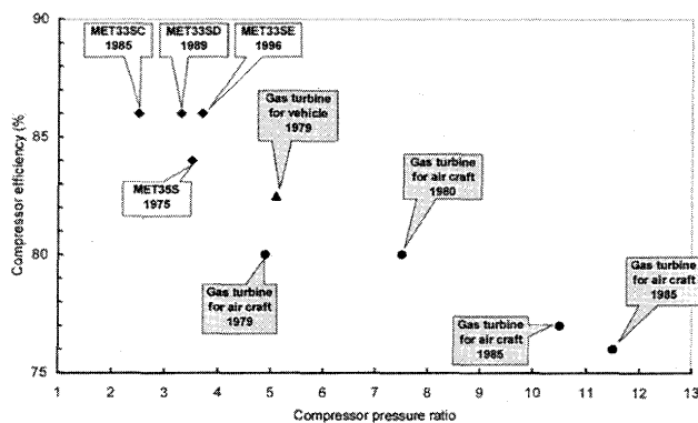
図9 単段コンプレッサの圧力比と効率
