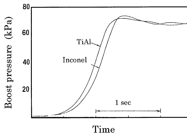
図 11 過渡特性比較
