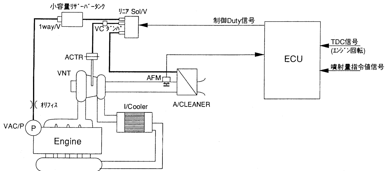
図9 VNターボ制御システムズ
