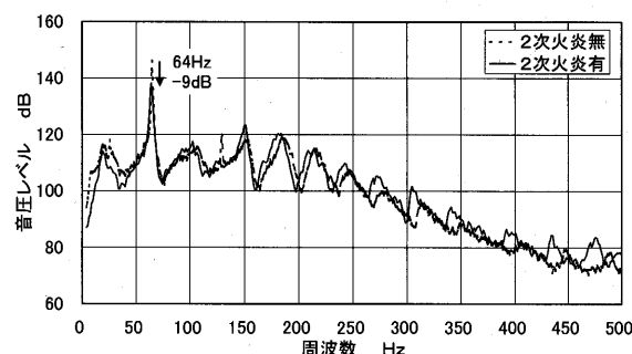
図4 音圧スペクトル(一定流量の場合)
