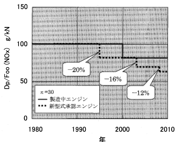
図1 ICAO による NOx 規制値の推移
