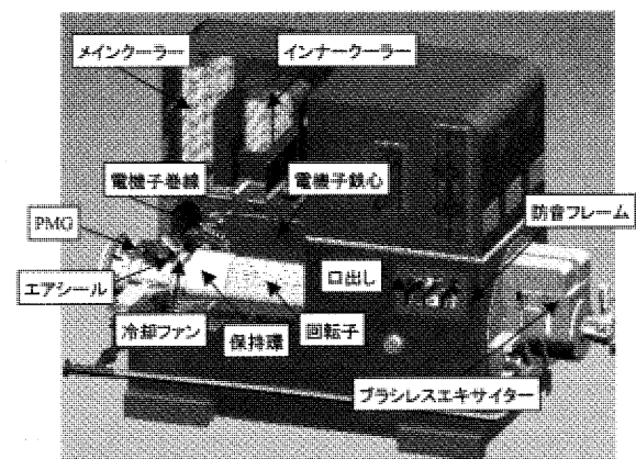
図1 高効率発電機 GH1550A (図は全閉型)
