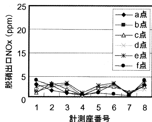
図5 出口 \text{NO}_x およびリーク \text{NH}_3 分布計測結果
