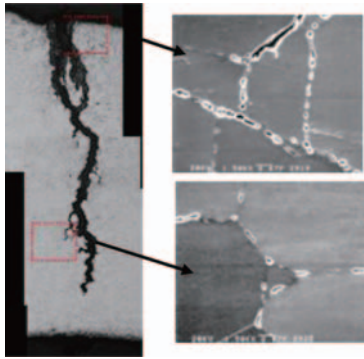
図4 き裂部断面の組織観察写真
