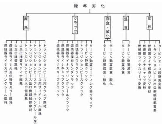
Fig. 3 ガスタービン高温部品の損傷形態
