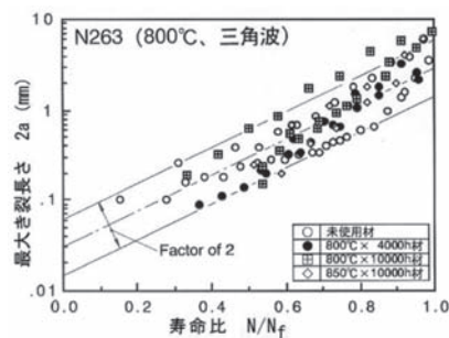
Fig.12 N263の最大き裂長さとして寿命比の関係
