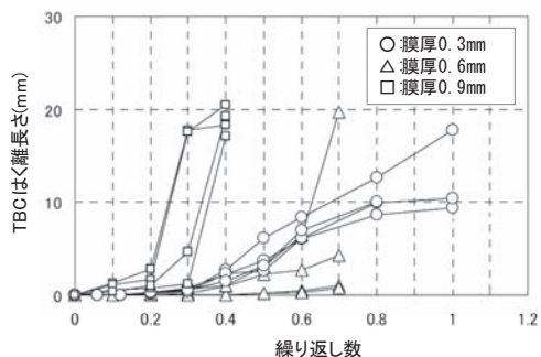
Fig.13 TBCの膜厚によるはく離進展挙動
