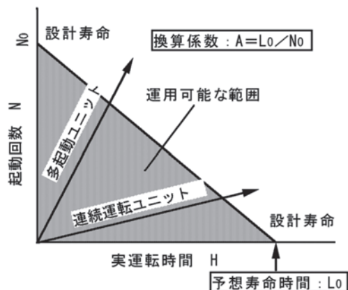
Fig. 4 高温部品寿命管理の概念
