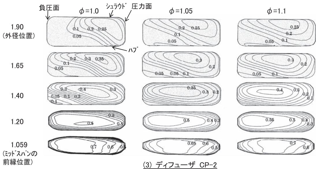
図12 ディフューザ流路断面内のマッハ数分布 R/R_2 はインペラ出口からの距離 (半径比)
