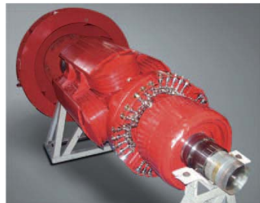
Fig. 4 Generator rotor
