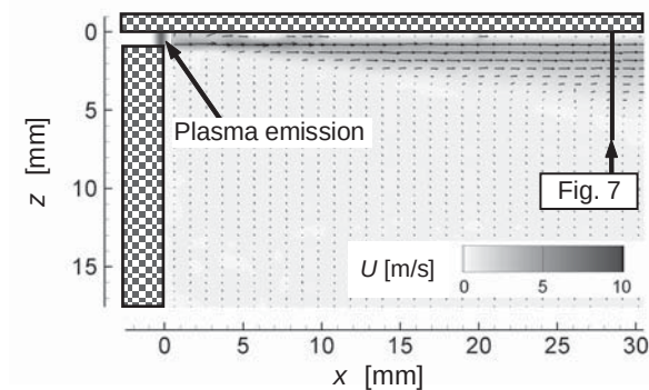
(d) Flow control ( f_p = 12 kHz)
