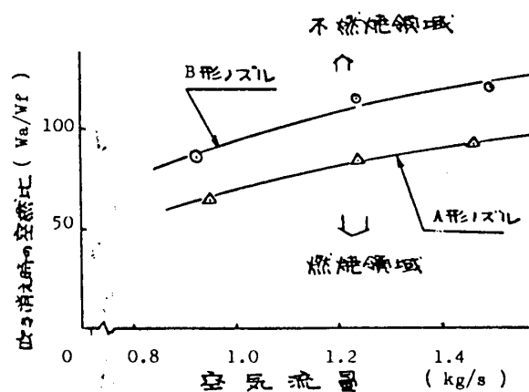
図9 吹き消え限界の比較
