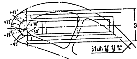
図8 前縁吹出模型
