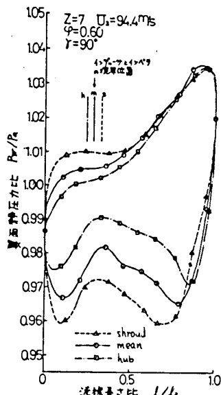
图6 静面静压力比分布
