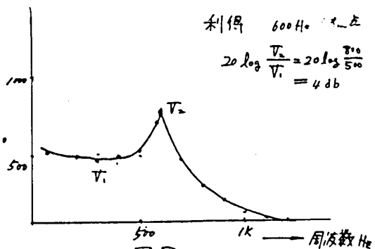
図 8 周波数特性
