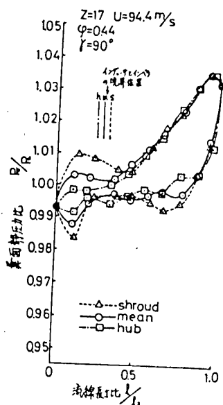
图12 静面静压力比分布
