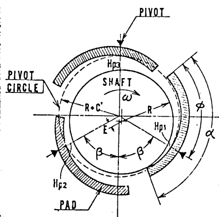
図2 空気軸受の模式図
