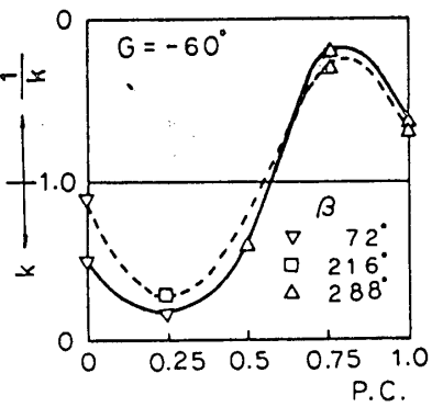
図5. 後退角60°の増速翼列のフロッタ限界と振り軸位置の内係
