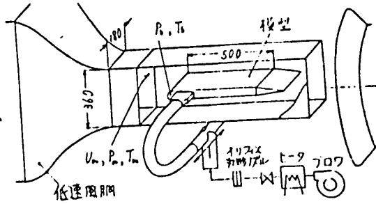
図7 実験装置
