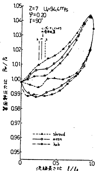
图8 静面静压力比分布
