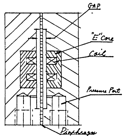
図4 Sensor部
