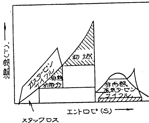
スタックロス (3) 排気燃焼サイクルのT-S線図。
