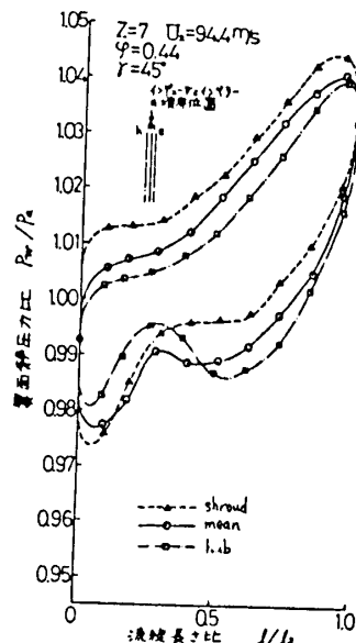
图10 静面静压力比分布
