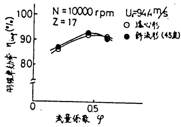
图5(b) 斜流形效率
