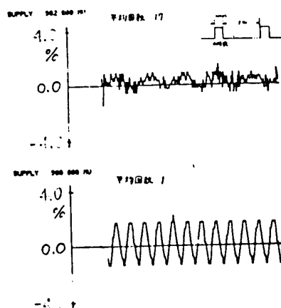
図13 高速AD変換器によるデータ
