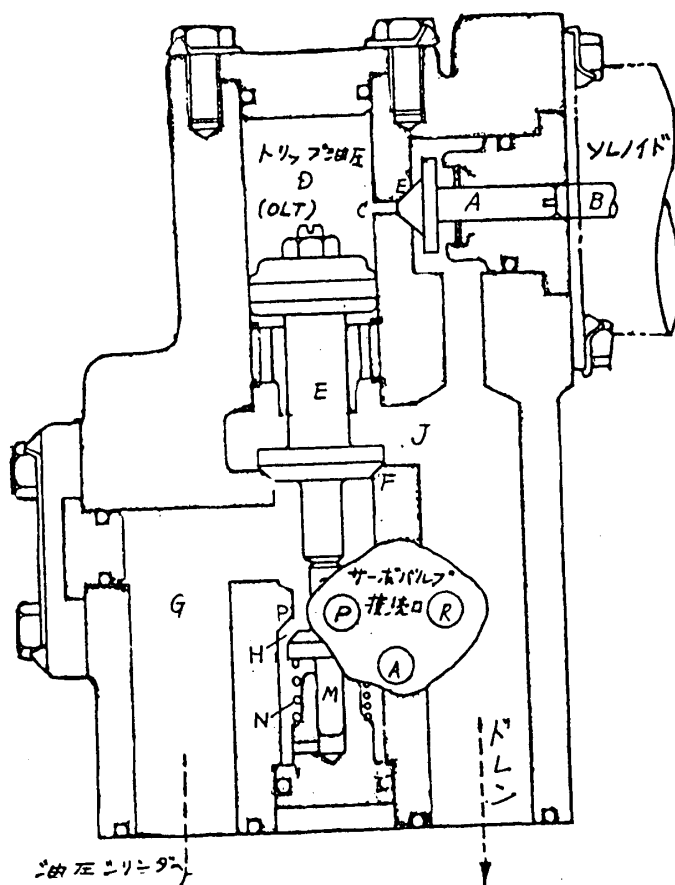
図9 ダンパバルブ断面図
