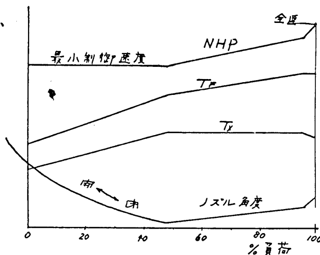
圖 6 NCE 控制線圖
