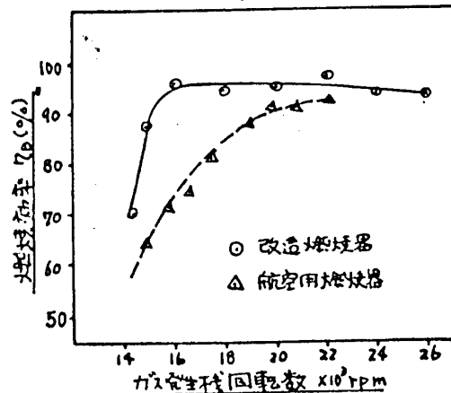
図4 ガスタービン特性
