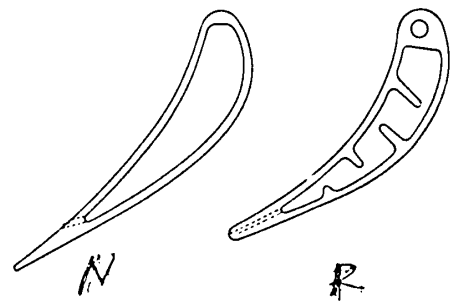
図2-4 翼形状図
