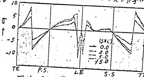
図16. 定肉厚翼の非定常熱応力分布(加熱)
