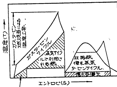
スタックロス (1) 単純排熱回収サイクル(助燃なし)のT-S線図。
