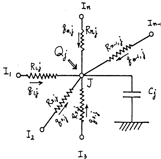
図 5-1 熱伝導モデル
