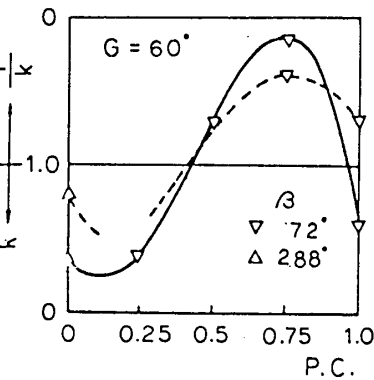
図6. 前進角60°の減速翼列のフロッタ限界と振り軸位置の内係
