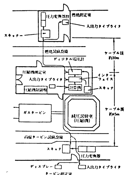
図2 計測系統図
