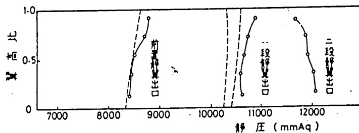
図 11 静圧分布
