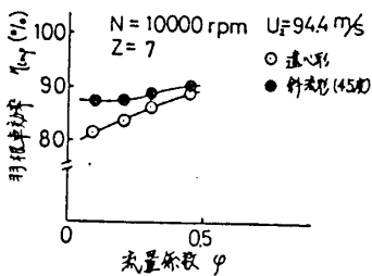
图5(a) 斜流形效率
