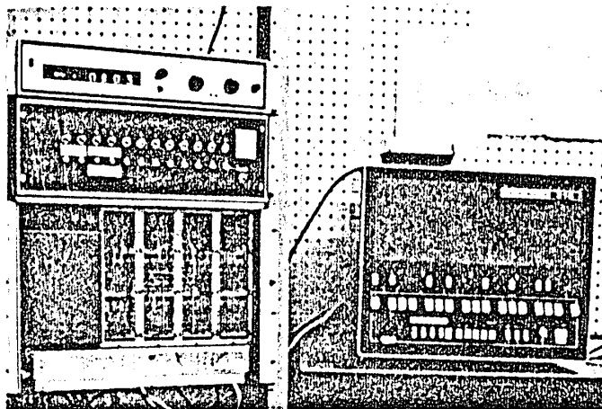
図3 端末側テ-タ集録装置
