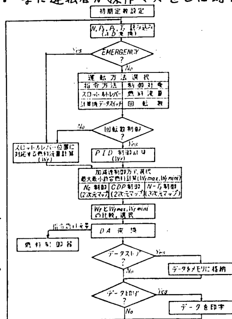
図4 ジェットエンジンの計算機制御流れ図
