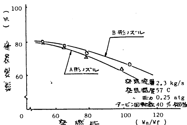
図10 タービン回転数40%相当の燃焼特性
