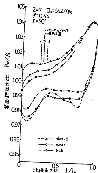
图7 静面静压力比分布
