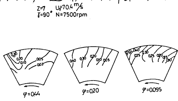
図14 羽根車内全圧力損失係数分布(遠心形)
