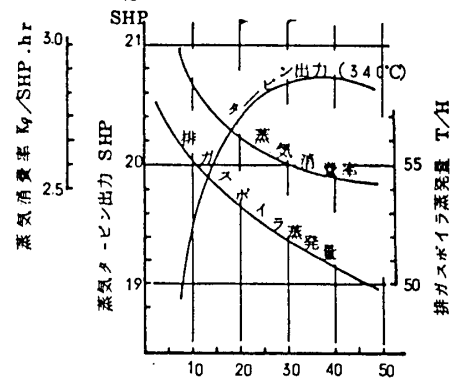
図-2 タービン入口蒸気圧力 %G 理想サイクル タービン出力
