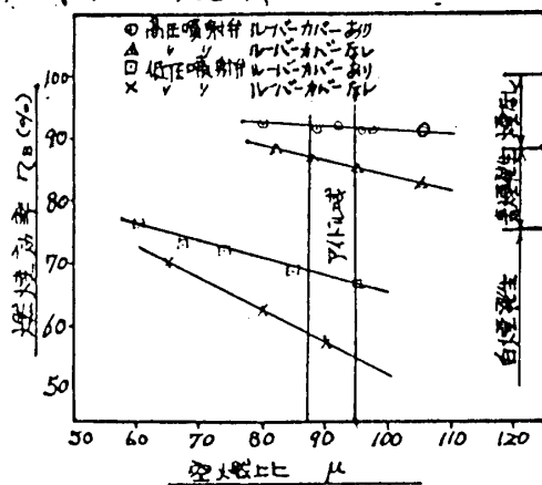
図3 着火特性
