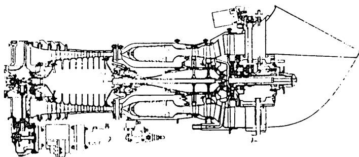
第2図 IM100-2G ガスタービン
